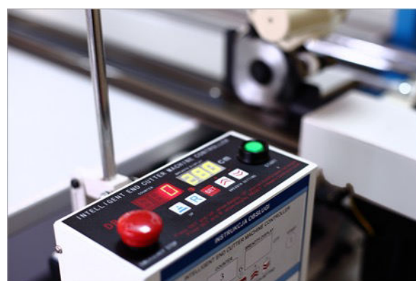
Panel sterujący odkrawacza w wersji Super i Super Plus. Licznik warstw, ustawianie długości cięcia i wysokość podnoszenia listwy.
