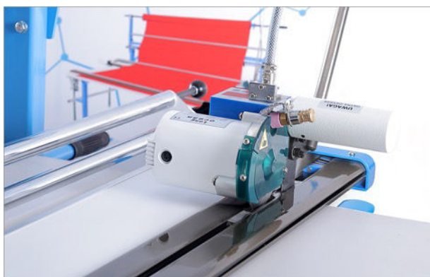
Odkrawacz ręczny w wersji Standard
